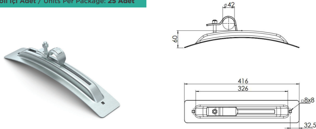
ÇAMURLUK KELEPÇESİ BÜYÜK GALVANİZ / BIG MUDGUARD'S CLAMP (ZP)
