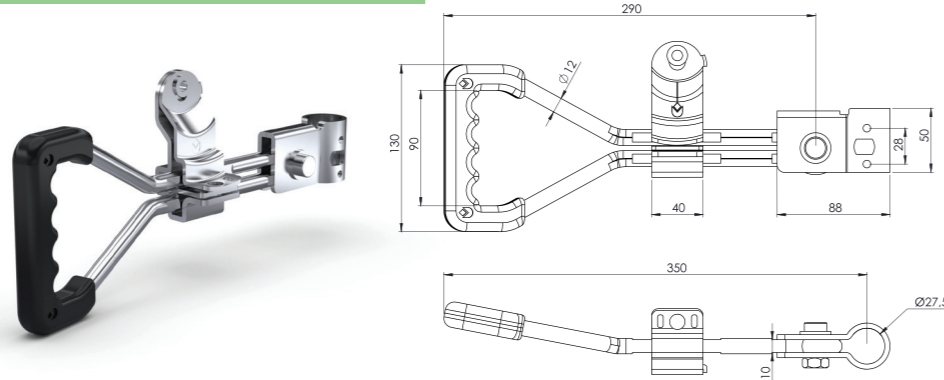
DELTA PLASTİKLİ MİL KOL TAKIM KROM - GALVANİZ Ø27 LEVER KIT Ø27 (SS) - (ZP)
