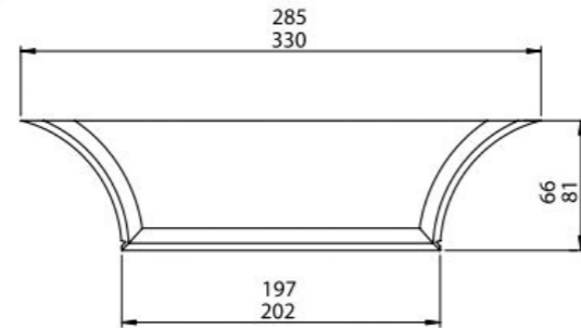
KÖŞELİ ETEK SACI / BRACKET
