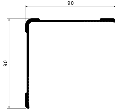
ALÜMİNYUM PROFİL / ALUMINIUM PROFILE
