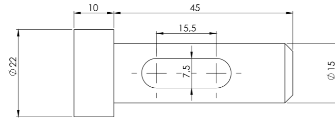
KALIP ERKEĞİ / MALE
