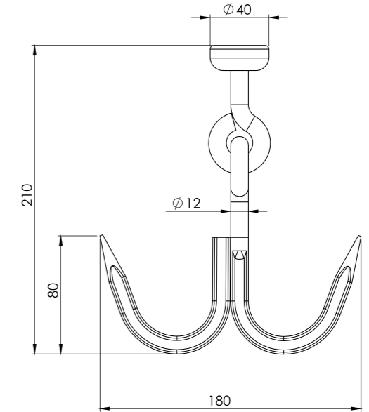
OYNAR BAŞLI ÇİFTLİ ET KANCASI KROM / MEAT HOOK (SS)
