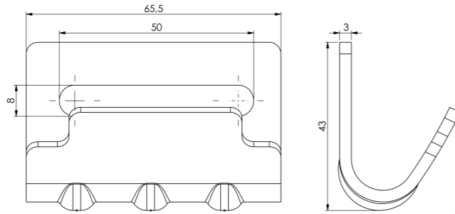
BRANDA TOKA KANCASI KROM - GALVANİZ TARPAULIN BUCKLE HOOK (SS) - (ZP)
