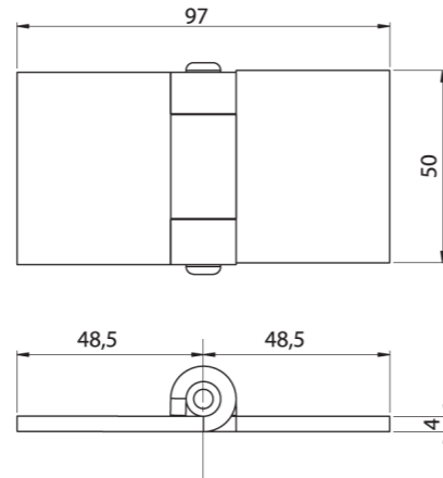
YAPRAK MENTEŞE 50MM / HINGE
