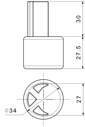
ADAPTÖR ÜST / ADAPTOR TOP
