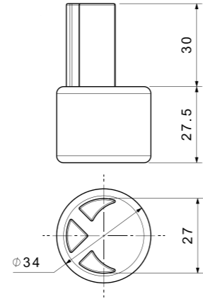
ADAPTÖR ALT / ADAPTOR BOTTOM
