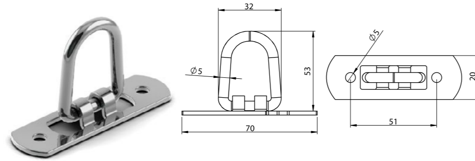
BRANDA KANCASI OYNAR BAŞLI GALVANİZ / TARPAULIN HOOK
