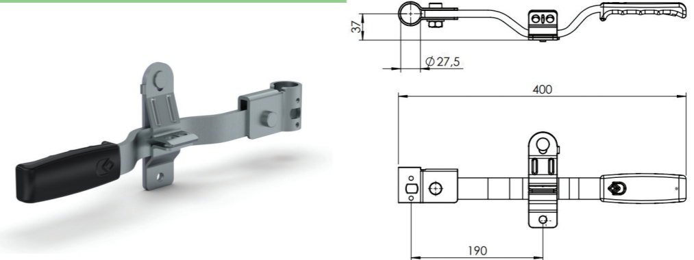
DÜZ PLASTİKLİ KOL TAKIM KROM - GALVANİZ Ø27 LEVER KIT Ø27 (SS) - (ZP)
