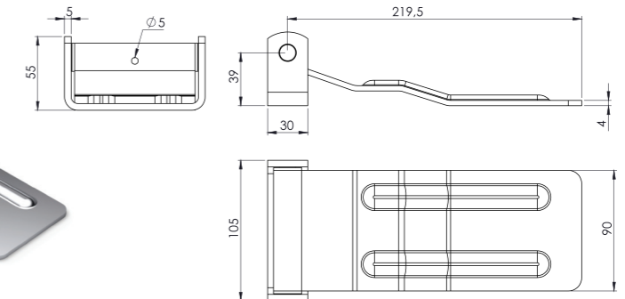
KAYNAK BAĞLANTILI MENTEŞE KAPLAMASIZ - GALVANİZ RAW - HINGE (ZP)
