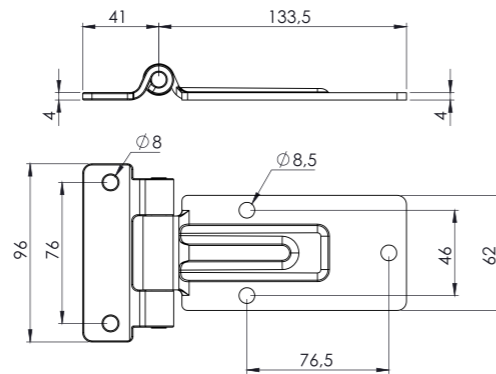
KÜÇÜK YAN KAPI MENTEŞESİ KROM - GALVANİZ SIDE DOOR HINGE (SS) - SIDE DOOR HINGE (ZP)
