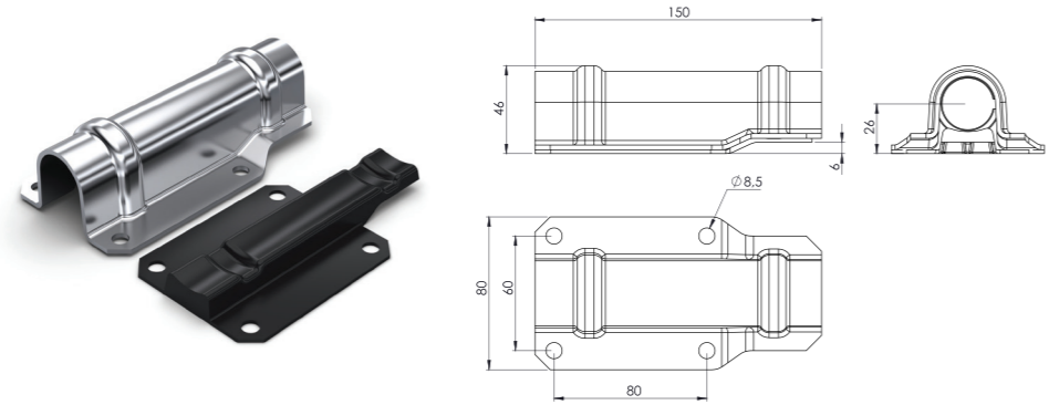
UNITNOVA EKO BÜYÜK BORU YUVASI KROM Ø27 UNITNOVA BIG GUIDE PLATE Ø27 (SS)
