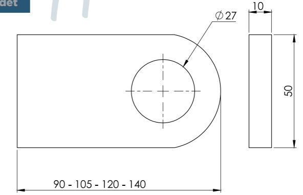
LAMA 50x9 - 50x10,5 - 50x12 - 50x14 / BRACKET
