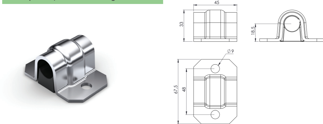
UNITNOVA BORU YUVASI KROM Ø16 / UNITNOVA GUIDE PLATE Ø16 (SS)
