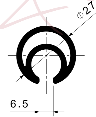
ALÜMİNYUM BORU / ALUMINIUM PIPE
