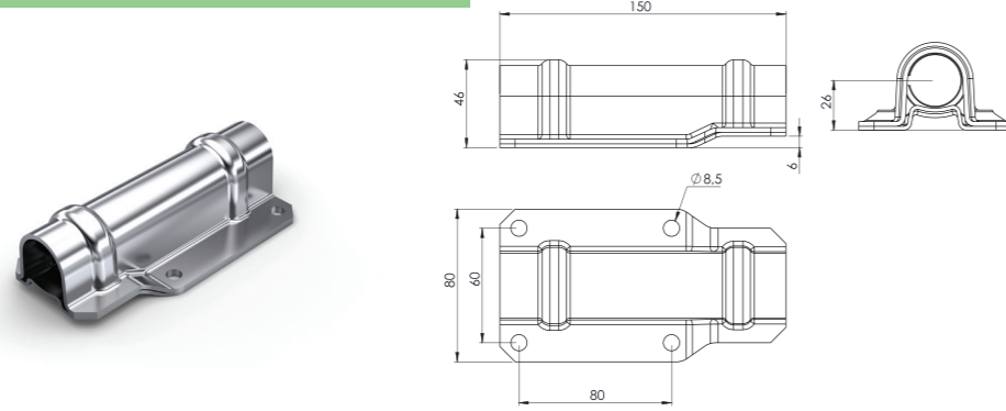
UNITNOVA BÜYÜK BORU YUVASI KROM Ø27 UNITNOVA BIG GUIDE PLATE Ø27 (SS)
