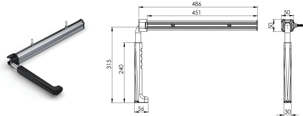
ALÜMİNYUM ARKA KAPI TUTAMAĞI / DOOR HOLDER (ALUMINIUM)
