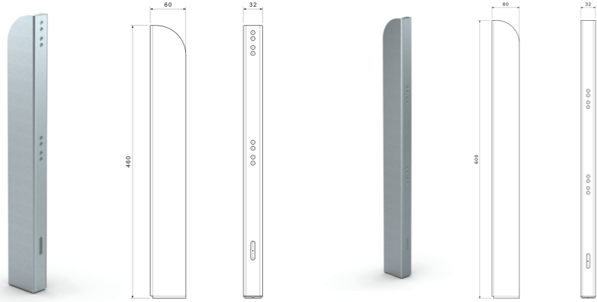
KAYAR BABA DEPOT SACI 462MM VE 600MM KATAFOREZLİ VE GALVANİZLİ SLIDING PILLAR SLAT STOWAGE 462MM & 600MM (ZINC+KTL)
