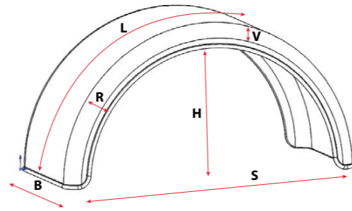
ÜSTÜ DÜZ BEYAZ ÇIZGİLİ ÇAMURLUK FLAT-TOP PLASTIC MUDGUARD WITH WHITE LINE
