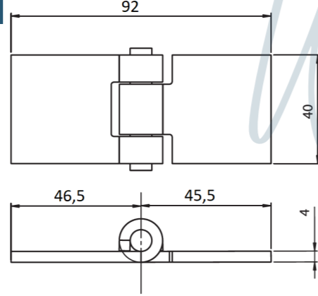
YAPRAK MENTEŞE 40MM / HINGE
