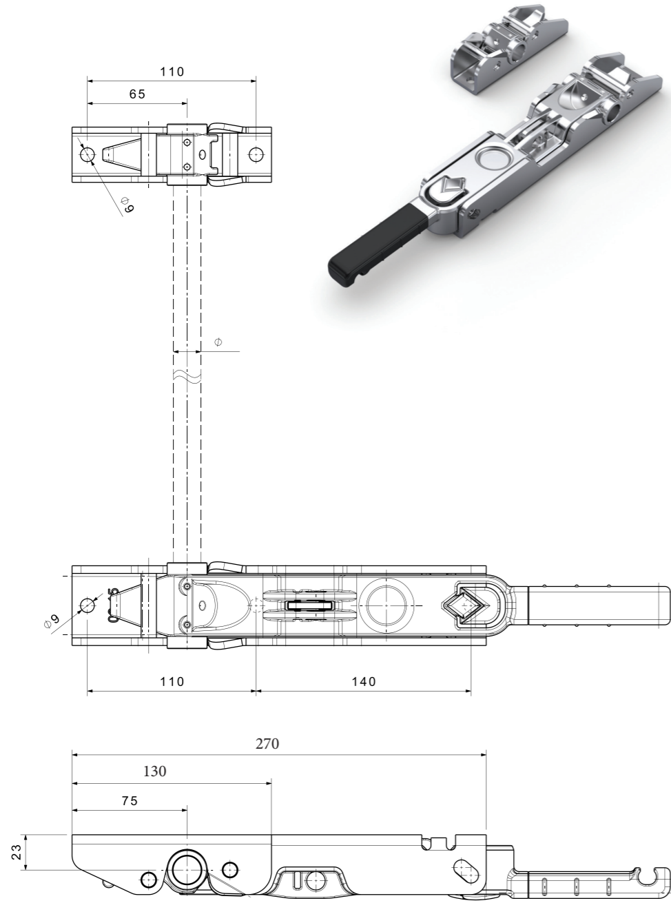
GİZLİ SİSTEM ARKA KAPI KİLİDİ (ÇİNKO+GEOMET) REAR DOOR FASTENER
