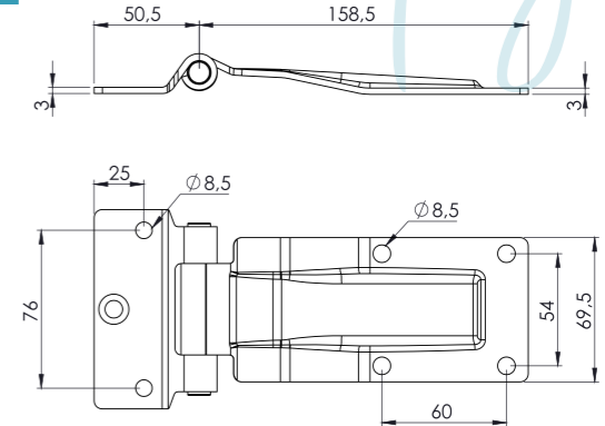
YAN KAPI MENTEŞESİ KROM - GALVANİZ SIDE DOOR HINGE (SS) - SIDE DOOR HINGE (ZP)
