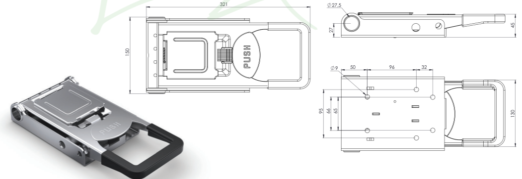
BÜYÜK DIŞTAN KİLİT KROM Ø27 - GALVANİZ Ø27 BIG PUSH HANDLE LOCK WITH KEY Ø27 (SS) - Ø27 (ZP)
