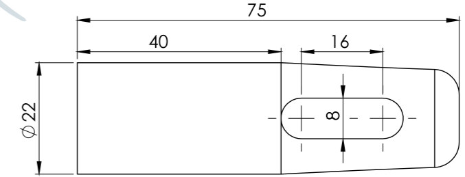
UZUN İLAVE ERKEĞİ / MALE
