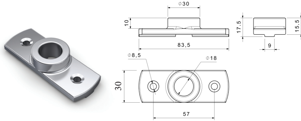
GİZLİ SİSTEM ÜST PARÇASI (ÇİNKO+GEOMET) - (GALVANİZLİ) REAR DOOR LOCK TOP BRACKET
