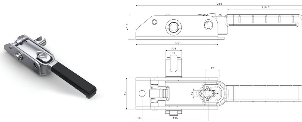
BRANDA GerdİRME MEKANİZMA APARATI TİP-1 U ADAPTÖRLÜ RATCHET TYPE 1
