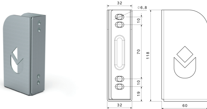
KAYAR BABA LALE LOGOLU TAHTALIK KATAFOREZLİ - GALVANİZLİ SLIDING PILLAR NEVPA LOGO SLAT STOWAGE -ZINC
