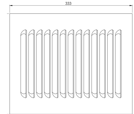
PANJUR ALUMİNYUM - KROM - GALVANİZ VENTILATION HATCH (ALUMİNYUM) - (SS) - (ZP)
