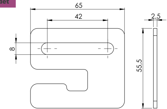
BRANDA TOKA E TİPİ KANCASI KROM - GALVANİZ TARPAULIN BUCKLE TYPE E HOOK (SS) - (ZP)
