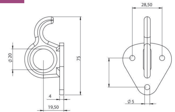
DORSE DÖVME KANCA GALVANİZ / RİNG (ZP)
