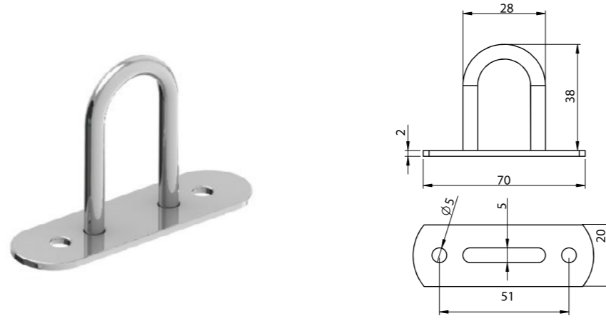
BRANDA KANCASI GALVANİZ / TARPAULIN HOOK
