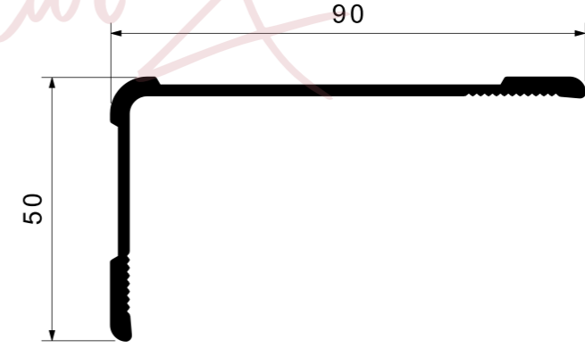
ALÜMİNYUM PROFİL / ALUMINIUM PROFILE
