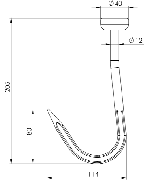
TEKLİ ET KANCASI KROM / MEAT HOOK (SS)
