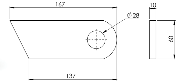
LAMA 60x10,5 / BRACKET
