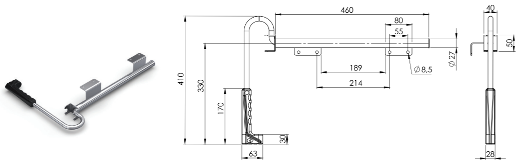
ARKA KAPI TUTAMAĞI DEVE BOYNU / DOOR HOLDER (ZP)
