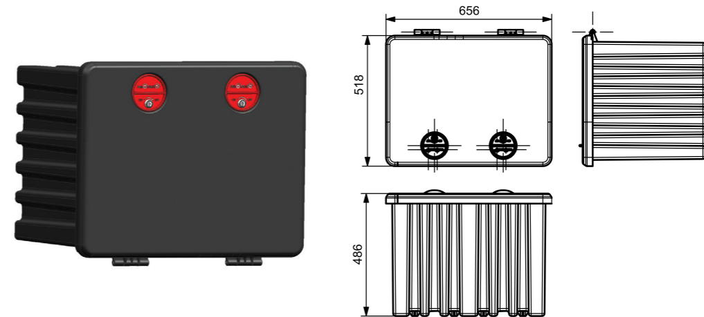
TAKIM DOLABI 60 / PRIMOGENITO TOOL BOX 60
