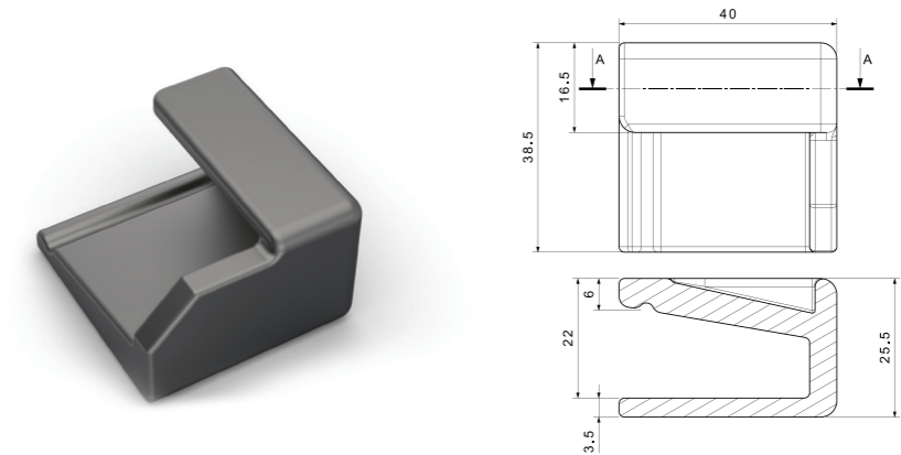
ALÜMİNYUM DİK KİLİT KARŞILIĞI ALUMINUM VERTICAL LOCKING SYSTEM - STRIKE PLATE
