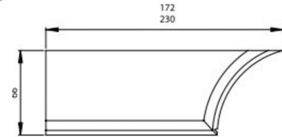
KÖŞELİ YARIM ETEK SACI / BRACKET
