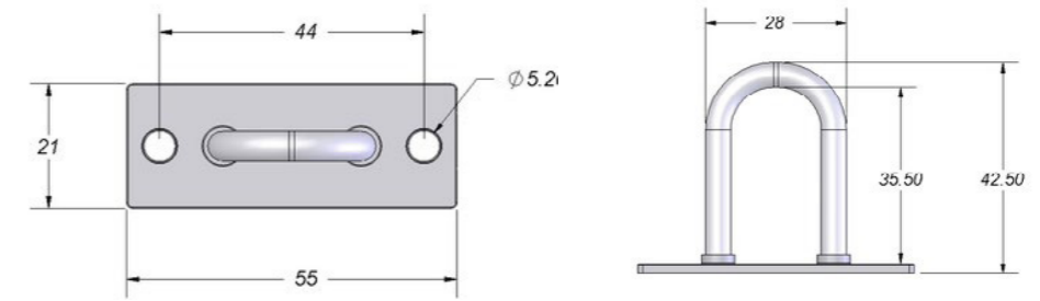
BRANDA KANCASI GALVANİZ / TARPAULIN HOOK
