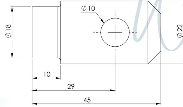
FATURALI TEK DELİKLİ ERKEK / MALE
