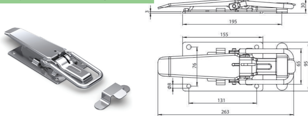
DÜZ DORSE KİLİDİ / FASTENER (ZP)
