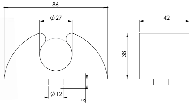
KÜÇÜK KAUÇUK BORU TAKOZU / RUBBER BUFFER
