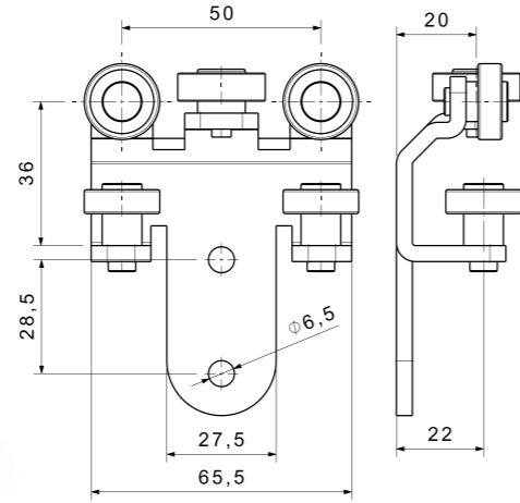
ACL PERDE MAKARASI / ACL CURTAIN ROLLER
